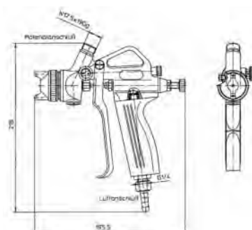
K HS-25 option gâchette longue + poignée
