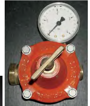
Manodétendeur 25 kg/h
